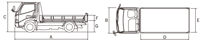
外形図
