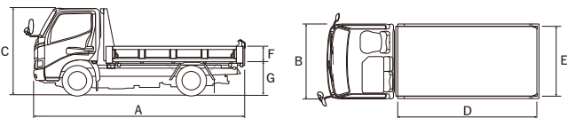
外形図
