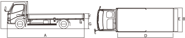
外形図
