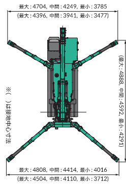
張出し寸法
