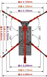
張出し寸法
