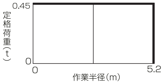
■ 定格荷重線図
