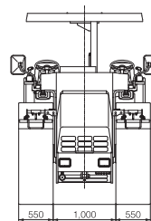
■外形寸法図(単位:mm) R2-1
